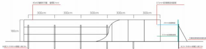
仿真草皮平面围挡立面施工图
