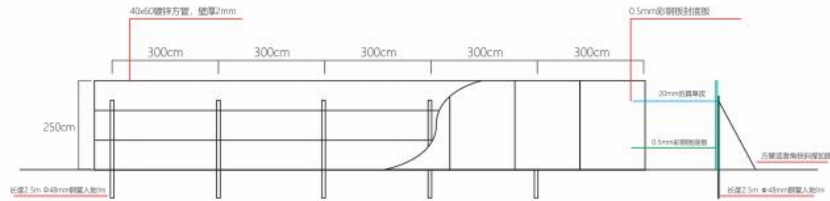
仿真草皮平面围挡立面施工图
