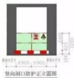
竖向洞口防护正立面图
