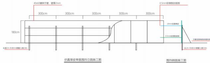
仿真草皮单面围挡立面施工图
