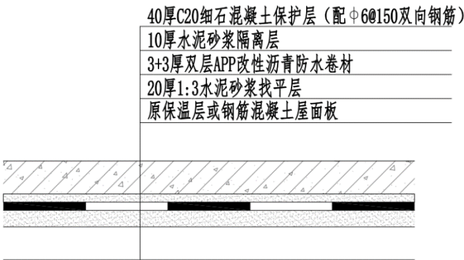
图 3.37 屋面防水做法示意图
