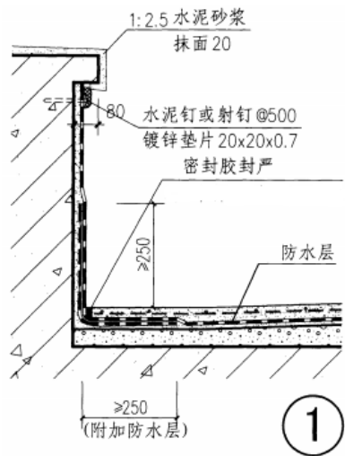
图 3.38 女儿墙防水做法示意图
