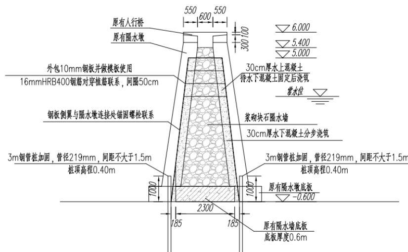
图 3.39 靠船墩维修加固示意图
