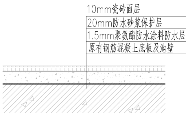
图 3.36 水池内壁防水做法示意图
