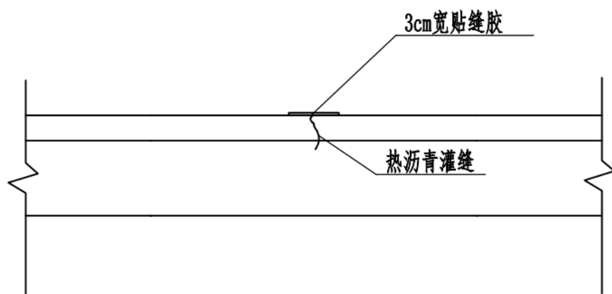
图 3.35 路面轻微开裂部位做法
