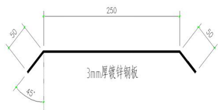
图七 纵向施工缝镀锌钢板止水带详图
