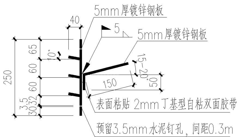
镀锌止水钢板大样 1:10
