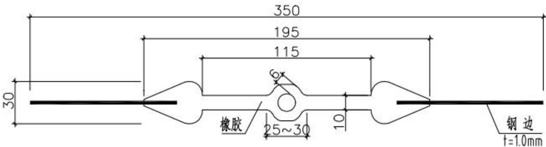
图一 中埋式中孔型钢边橡胶止水带详图
