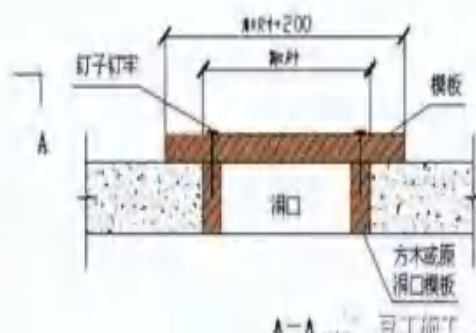
A-A 剖面图
