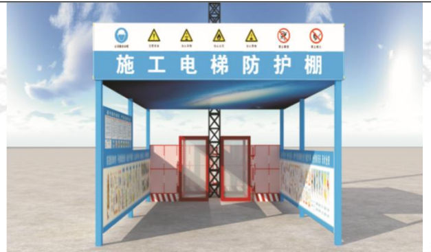
图 37 施工电梯防护棚
