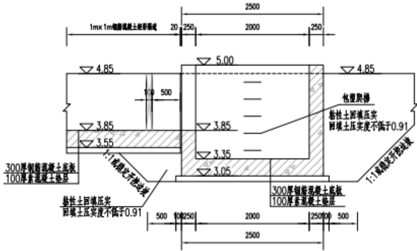
图 3.4.10-2 出水井 1-1 剖面图
