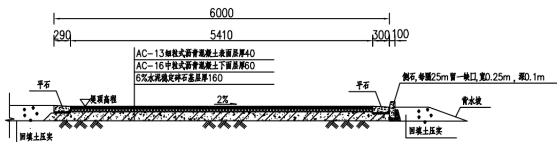
图 9-1 堤顶路面开裂部位修复做法
