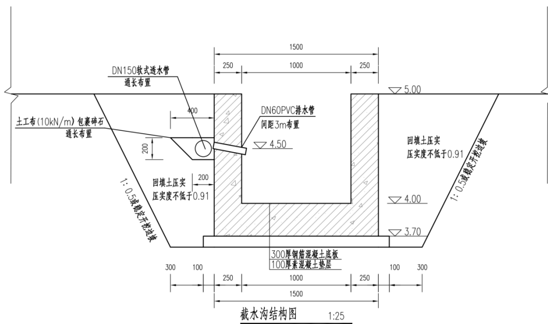
图 10-1 截水沟结构图
