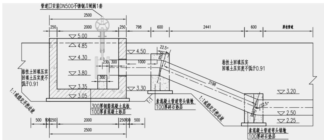
图 3.4.10-3 出水井 2-2 剖面图
