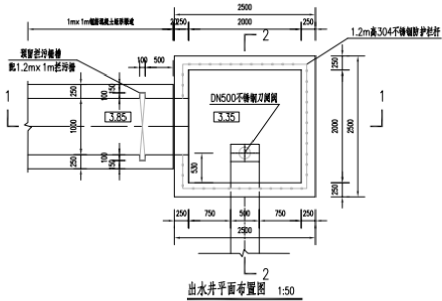
图 3.4.10-2 出水井平面图
