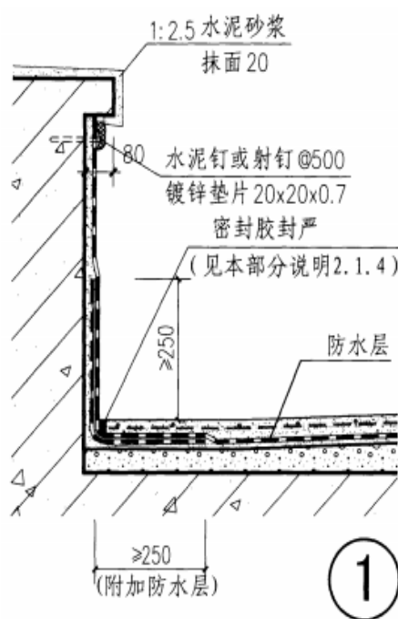
图 2-1 女儿墙卷材做法
