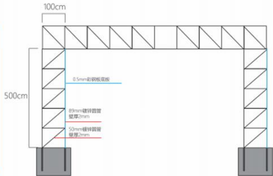
门楼立柱施工图
