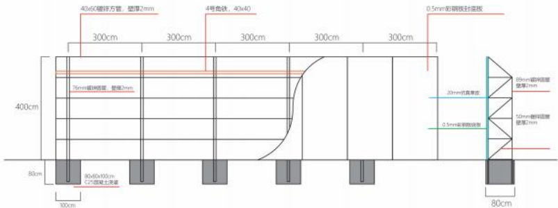
仿真草皮单面围挡立面施工图
