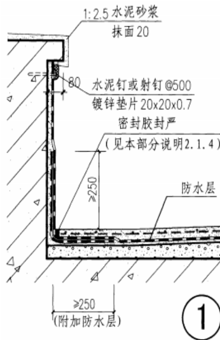
女儿墙卷材做法
