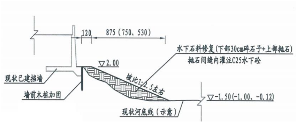
挡墙前侧护坡修复做法
