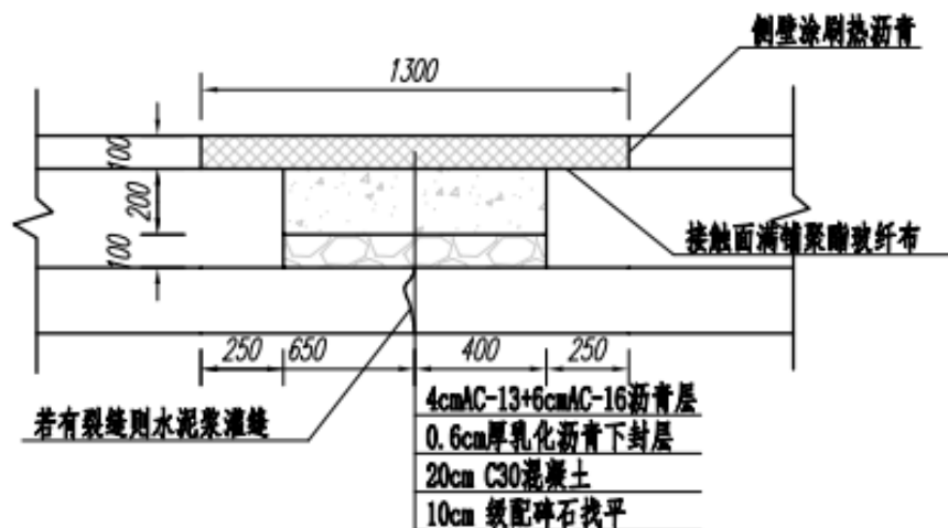
堤顶路水稳层损坏严重部位修复做法
