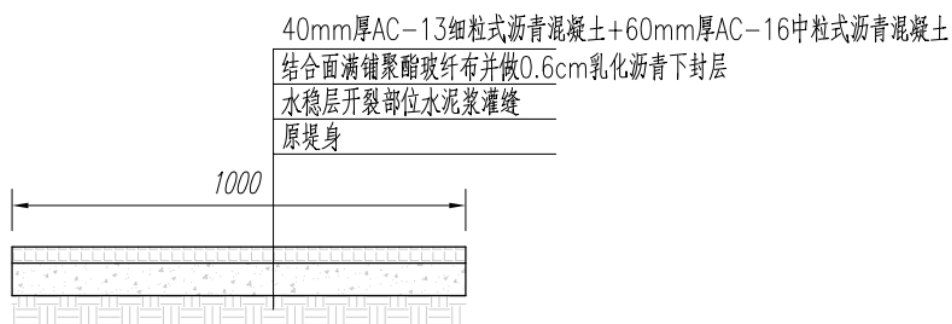
堤顶路面开裂部位修复做法
