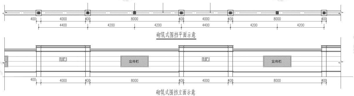
图 12 新中式风格砌筑式围挡尺寸
