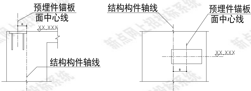
预埋件在构件施工图中的定位表示方法
