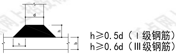
手工电弧焊的构造要求
