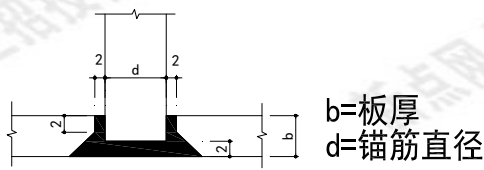
穿孔塞焊的构造要求
