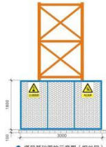
● 塔吊基础面防护示意图（铁丝网）
