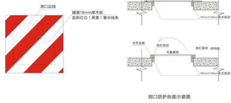
● 洞口防护示意图
