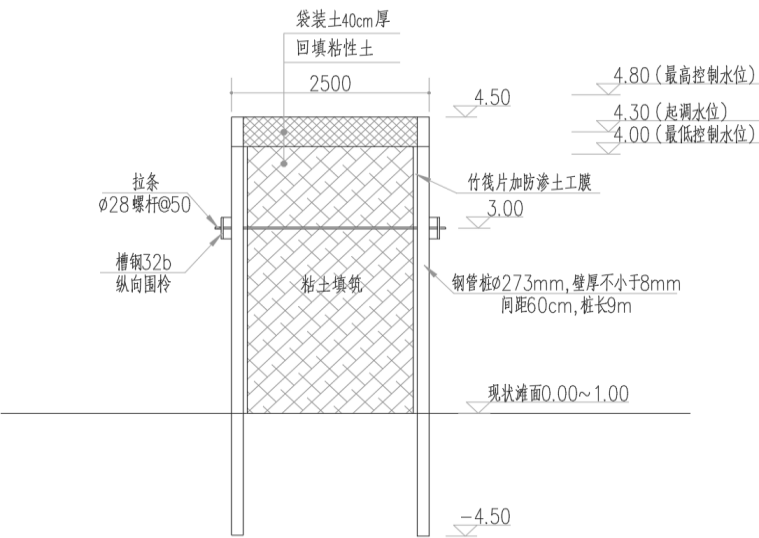
图 4.3-1 桩土复合围堰
