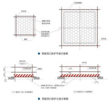
预留洞口防护示意图
