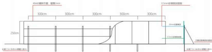
仿真草皮单面围挡立面施工图
