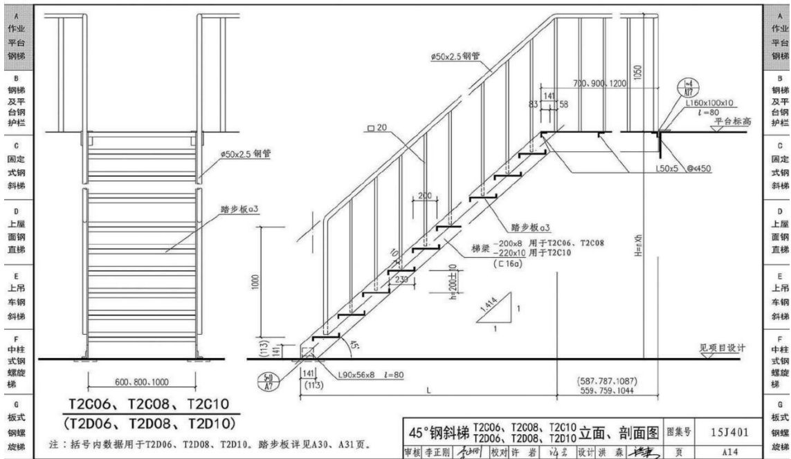
图 3.4.8.1-1 45° 钢斜梯做法立面、剖面图
