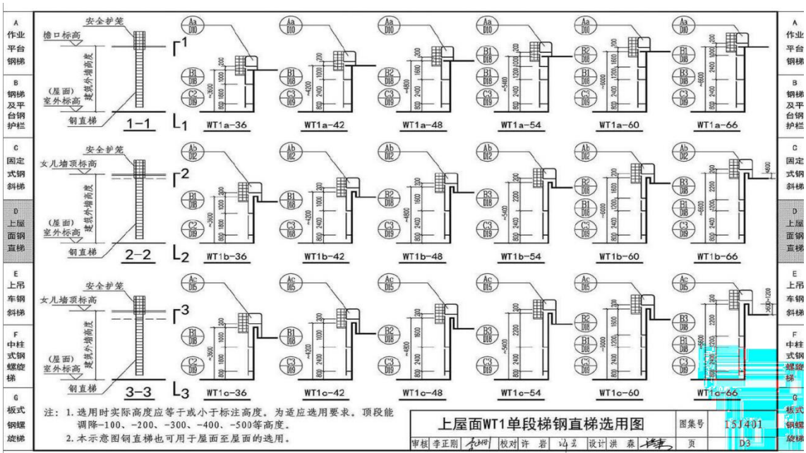
图 3.4.8.2-1 丁横河枢纽 5#机组检修井 WT1a-66 型直梯做法图
