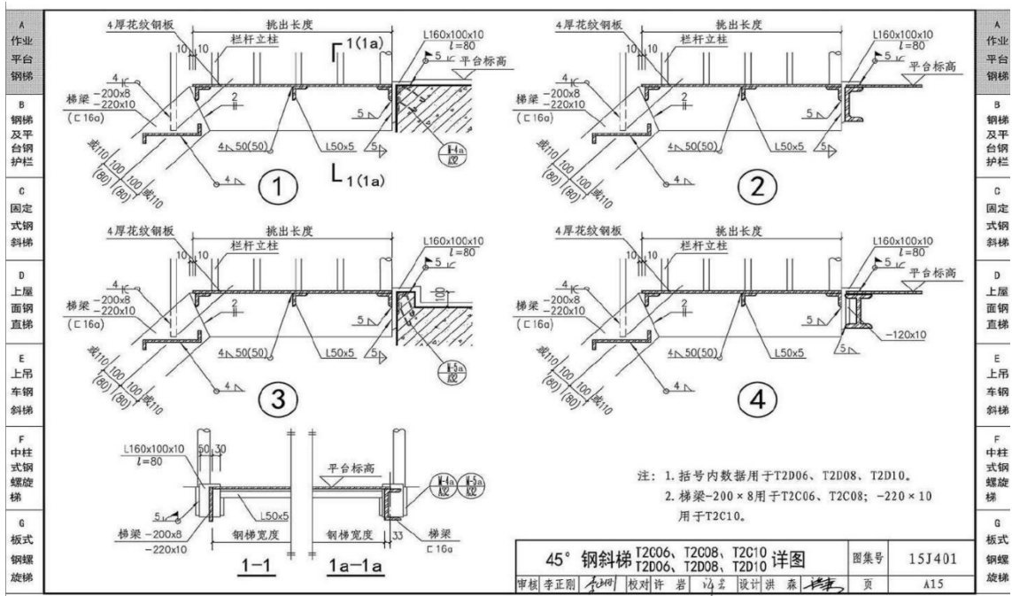
图 3.4.8.1-2 45° 钢斜梯做法详图
