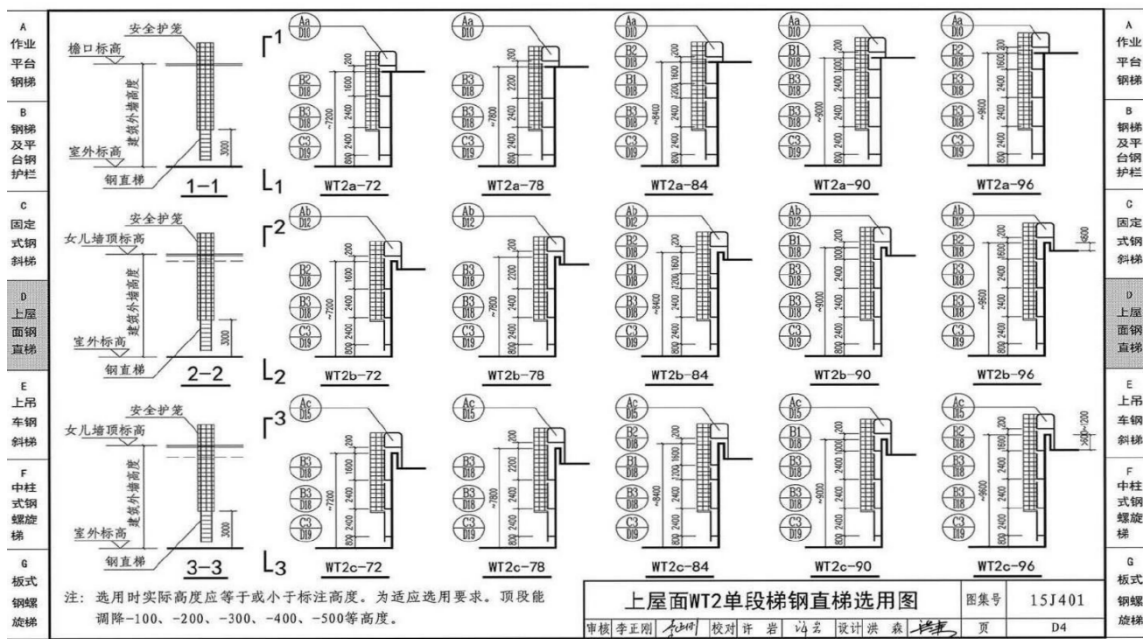
图 3.4.8.2-2 大运河东枢纽泵房屋面 WT2b-72 型直梯做法图
