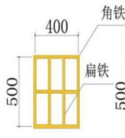
侧图1
