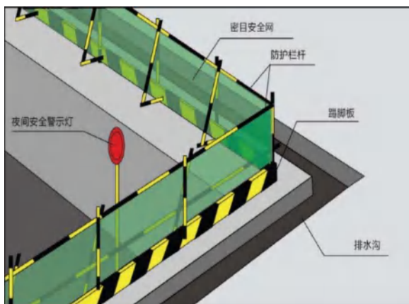
定型化防护栏
