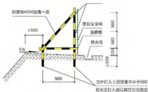
基坑临边防护剖面图 / 单位 mm
