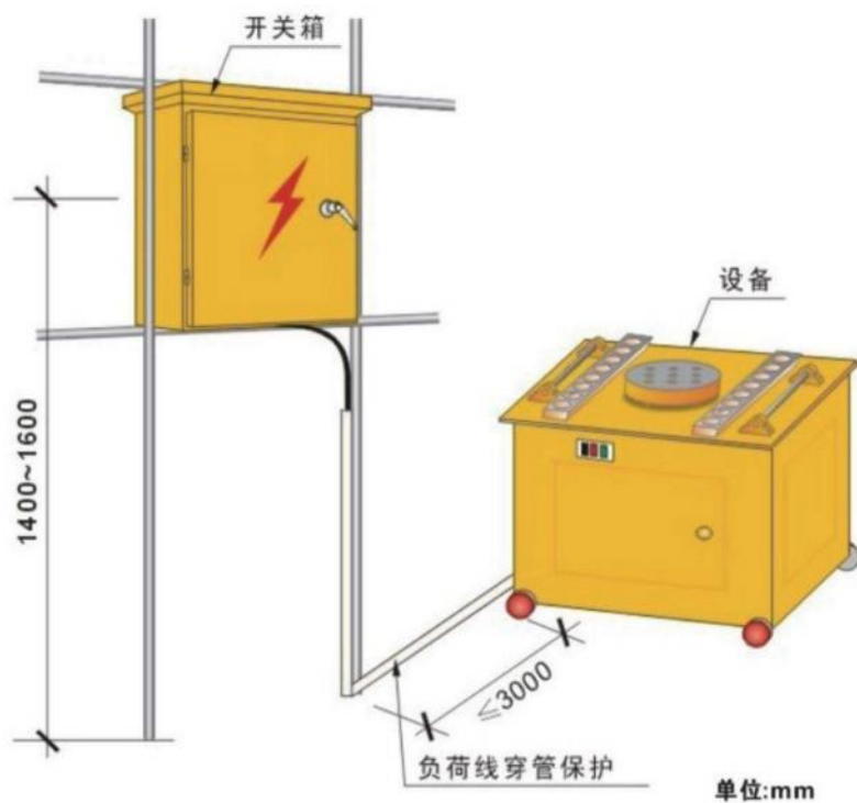
设备与电源距离图
