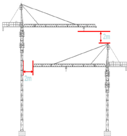
塔吊安全距离
