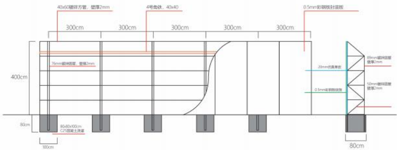
仿真草皮单面围挡立面施工图
